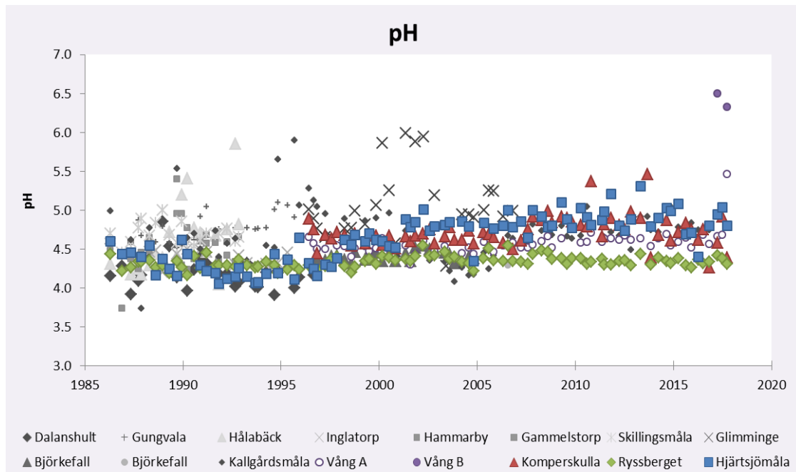
Figur 16. En sammanställning av alla förekommande mätningar av pH i markvattnet i länet. Markvattnet provtas tre gånger årligen, före, under och efter växtsäsongen. Vissa provtillfället saknas när det varit torrt i marken. Aktiva mätplatser visas med färgade symboler och avslutade mätplatser visas med symboler i grått och svart.
