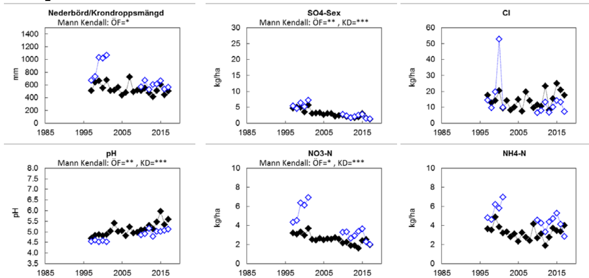
- ◆ - Krondropp (KD) Figur B1.5. Årliga värden (hydrologiskt år) för depositionen via krondropp och över öppet fält vid Komperskulla, K 11. I figuren visas uppmätt nederbörd över öppet fält samt krondroppsmängder sedan mätstart. Vidare redovisas nederbördens och krondroppets pH, liksom deposition för ett urval av ämnen: sulfatsvavel utan havssaltsbidrag (SO 4 -S ex), klorid (Cl - ), nitratkväve (NO 3 -N) och ammoniumkväve (NH 4 -N). Trendanalys har genomförts med Mann-Kendall-analys. Signifikansnivåer anges, ovanför respektive diagram, i de fall där signifikanta trender påvisats. - ◇ - Öppet fält (ÖF)
