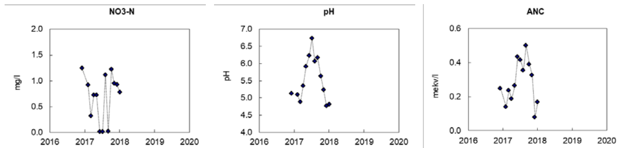
Figur B1.9. Bäckvattenkemi vid Vång, K 13A: nitratkväve ( \text{NO}_3\text{-N} ), pH och markvattnets syraneutraliserande förmåga (ANC).
