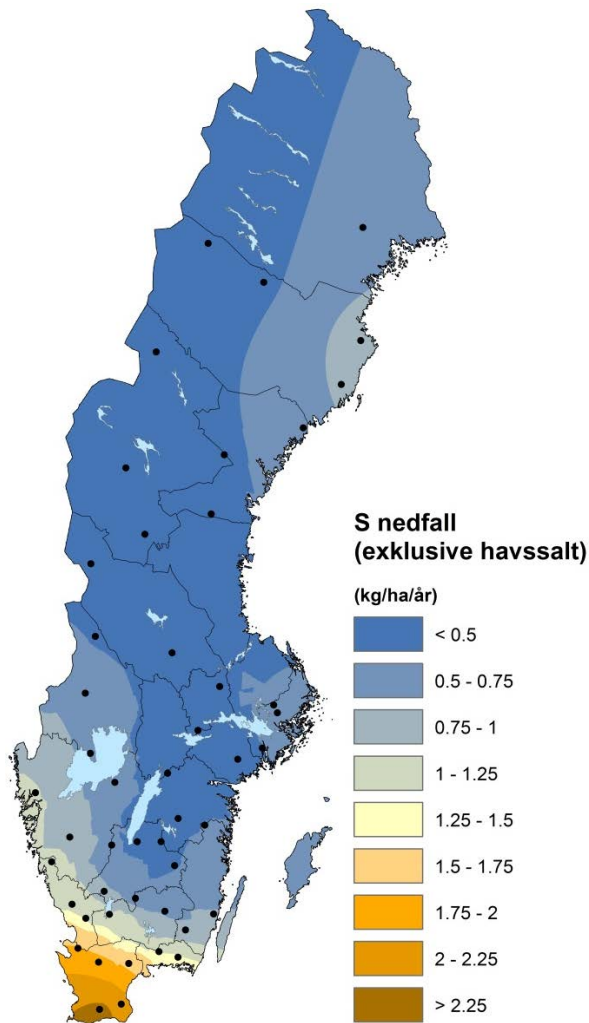
Figur 11. Svavelnedfall (exklusive bidraget från havssalt) under 2016/17 i krondroppet vid mätstationerna (gran och tall) inom Krondroppsnetet i Sverige.
