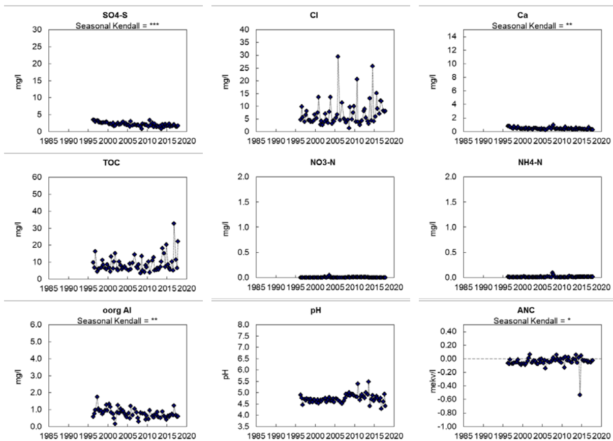
Figur B1.6. Markvattenkemi vid Komperskulla, K 11: sulfatsvavel (SO 4 -S), klorid (Cl - ), kalciumhalt (Ca 2+ ), totalt organiskt kol (TOC), nitratkväve (NO 3 -N), ammoniumkväve (NH 4 -N), oorganiskt aluminium (oorg Al), pH och markvattnets syraneutraliserande förmåga (ANC). Saknade värden innebär oftast att marken varit för torr. Trendanalys har genomförts med Seasonal-Kendall och signifikansnivåer anges, ovanför respektive diagram, i de fall där signifikanta trender påvisats.
