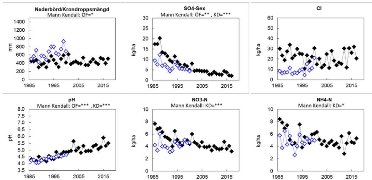
Figur B1.3. Årliga värden (hydrologiskt år) för depositionen via krondropp och över öppet fält vid Ryssberget, K 07. I figuren visas uppmätt nederbörd över öppet fält samt krondroppsmängder sedan mätstart. Vidare redovisas nederbördens och krondroppets pH, liksom deposition för ett urval av ämnen: sulfatsvavel utan havssaltsbidrag ( \text{SO}_4\text{-S ex} ), klorid ( \text{Cl}^- ), nitratkväve ( \text{NO}_3\text{-N} ) och ammoniumkväve ( \text{NH}_4\text{-N} ). Trendanalys har genomförts med Mann-Kendall-analys. Signifikansnivåer anges, ovanför respektive diagram, i de fall där signifikanta trender påvisats.
