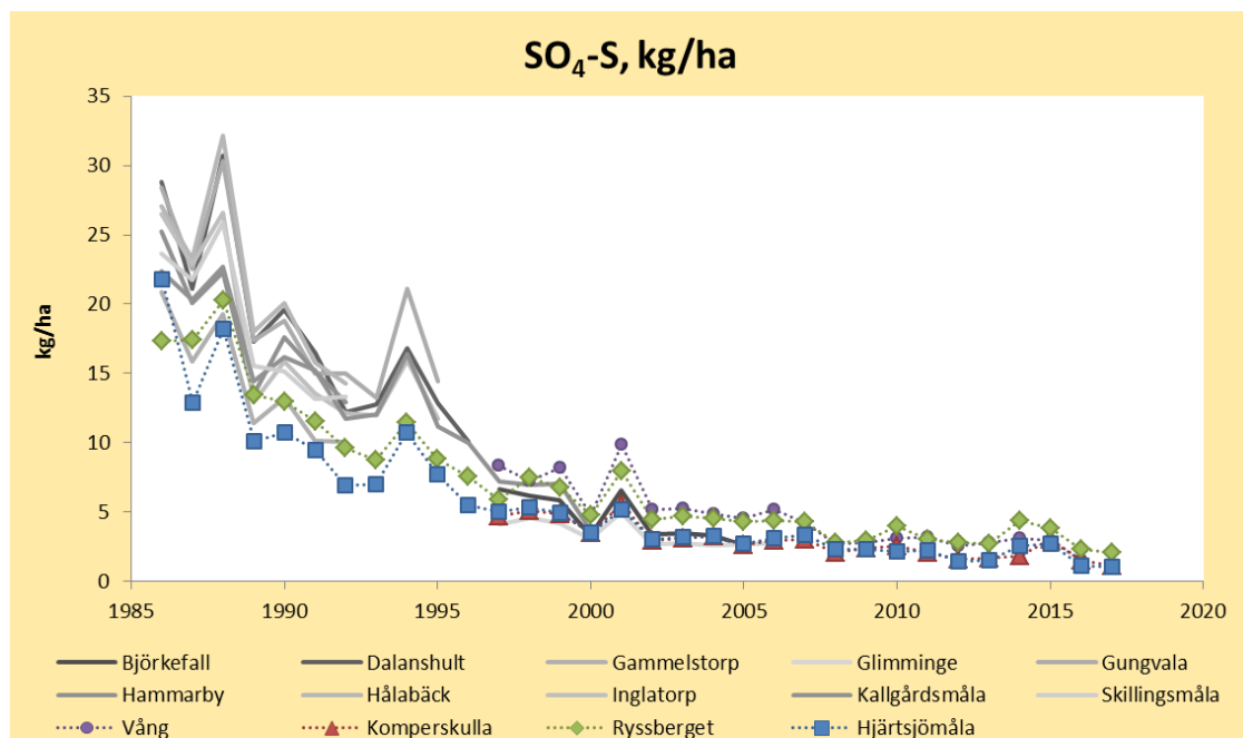
Figur 10. En sammanställning av alla förekommande mätningar av svavelnedfall (exklusive havssaltsbidrag) som krondropp i länet. Nedfallet mäts månadsvis och är summerat per hydrologiskt år. Aktiva mätplatser visas med färgade symboler och avslutade mätplatser visas med linjer i grått och svart.
