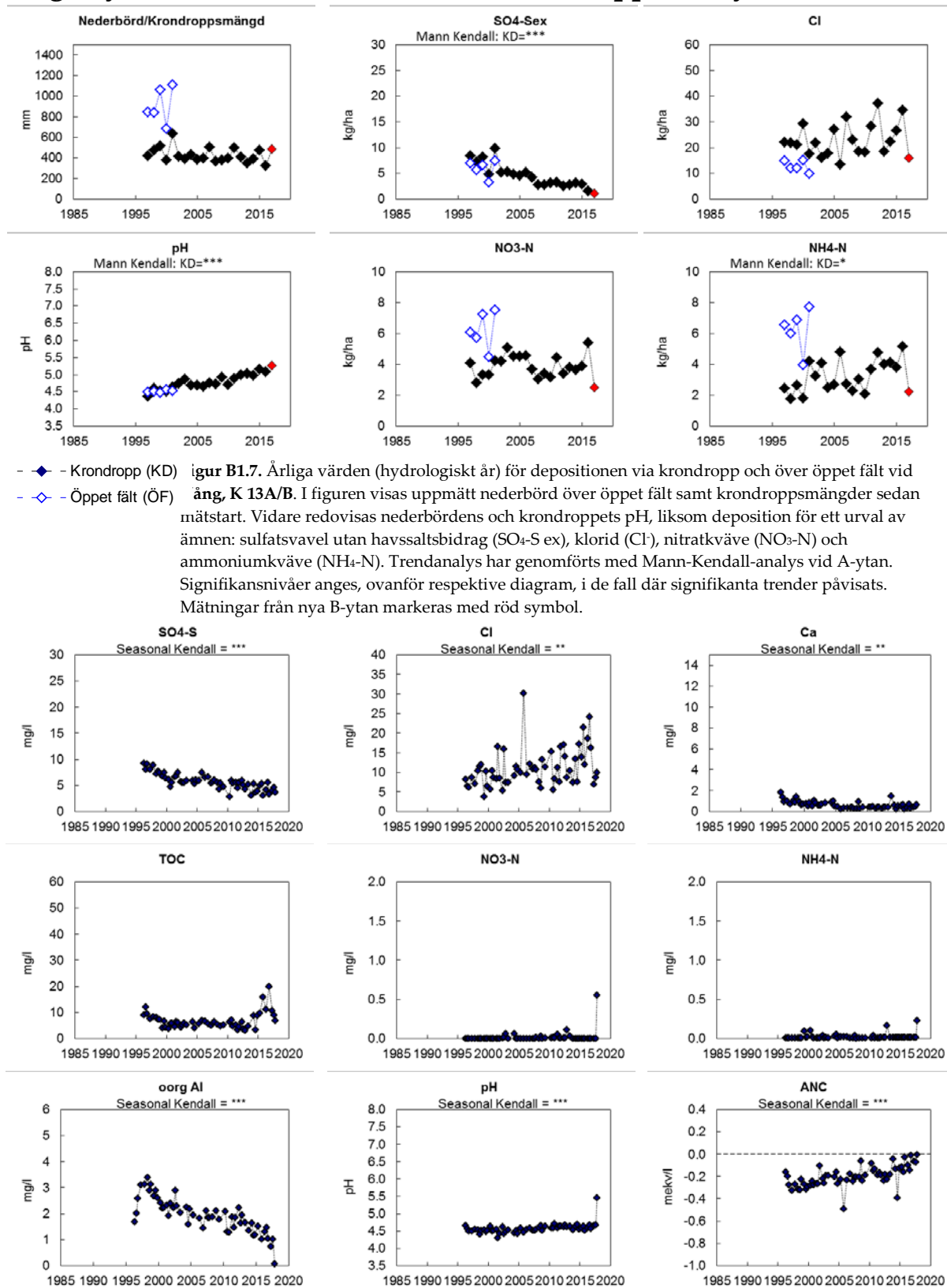
Figur B1.8. Markvattekemi vid Vång, K 13A: sulfatsvavel (SO 4 -S), klorid (Cl - ), kalciumhalt (Ca 2+ ), totalt organiskt kol (TOC), nitratkväve (NO 3 -N), ammoniumkväve (NH 4 -N), oorganiskt aluminium (oorg Al), pH och markvattnets syraneutraliserande förmåga (ANC). Saknade värden innebär oftast att marken varit för torr. Trendanalys har genomförts med Seasonal-Kendall och signifikansnivåer anges, ovanför respektive diagram, i de fall där signifikanta trender påvisats.
