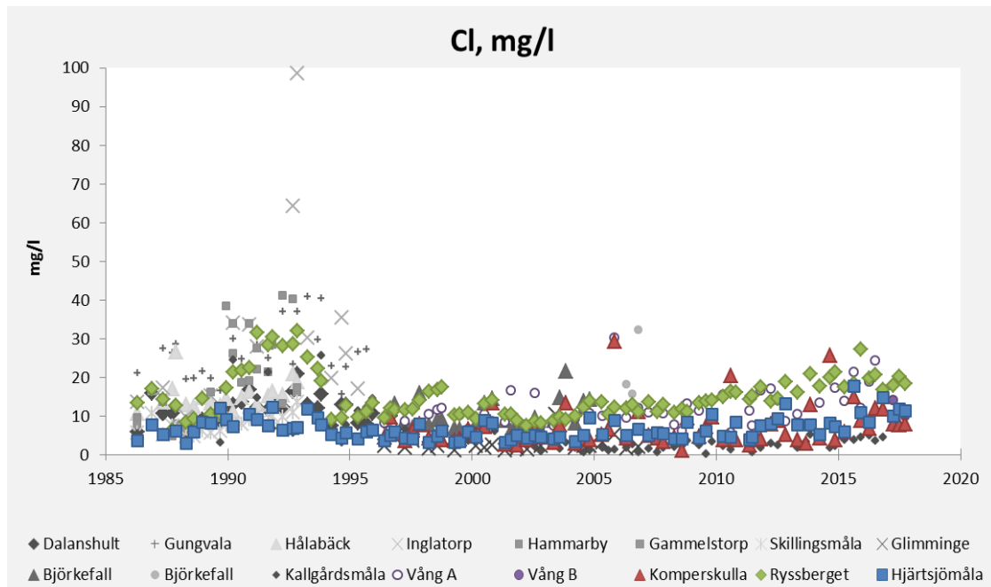
Figur 14. En sammanställning av alla förekommande mätningar av klorid i markvattnet i länet. Markvattnet provtas tre gånger årligen, före, under och efter växetsäsongen. Vissa provtillfället saknas när det varit torrt i marken. Aktiva mätplatser visas med färgade symboler och avslutade mätplatser visas med symboler i grått och svart.
