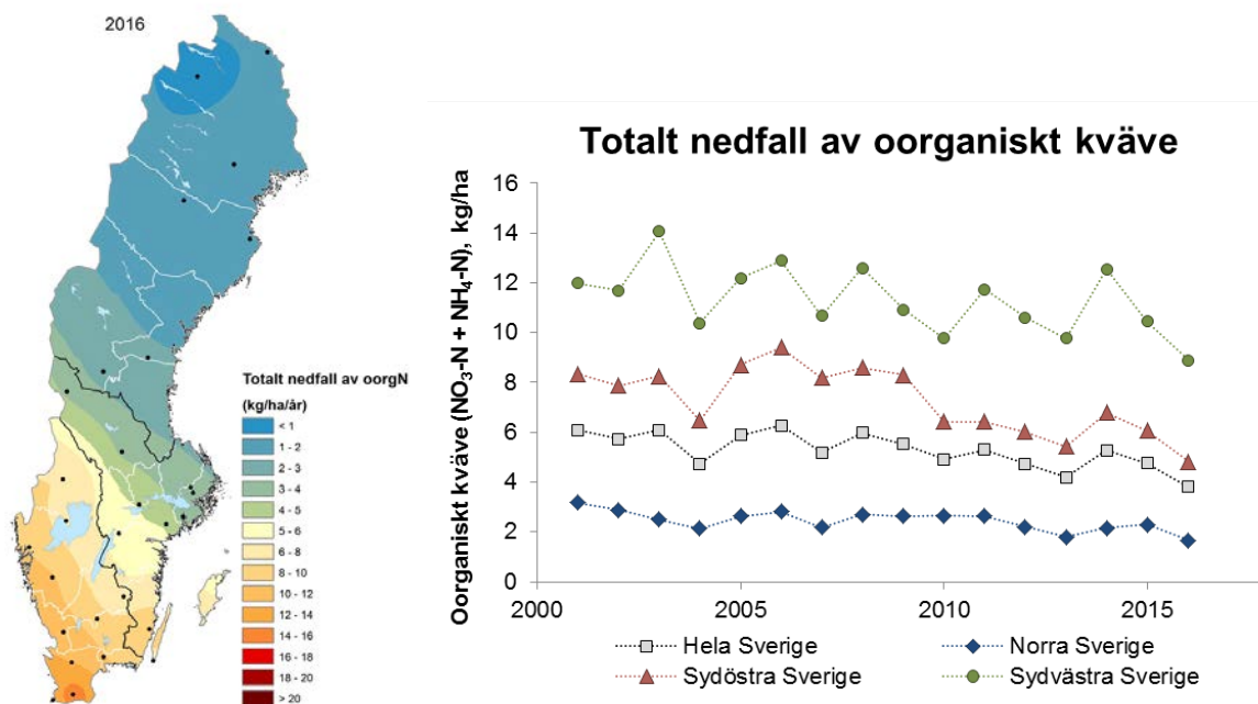
Figur 19. A. En karta över geografiskt interpolerade värden för totalt nedfall av kväve till barrskog för kalenderåret 2016. Svarta punkter indikerar mätplatser. Sverige är indelat i tre geografiska områden som används inom uppföljningen av miljökvalitetsmålen. Dessa områden används i figuren med tidsserier. B. Tidsserier för årligt nedfall av oorganiskt kväve (NO 3 -N + NH 4 -N) till barrskog för tre olika geografiska områden över Sverige, norra Sverige, sydöstra Sverige samt sydvästra Sverige. Beräkningarna inkluderar summan av torr- och våtdeposition och baseras på kalenderår.
