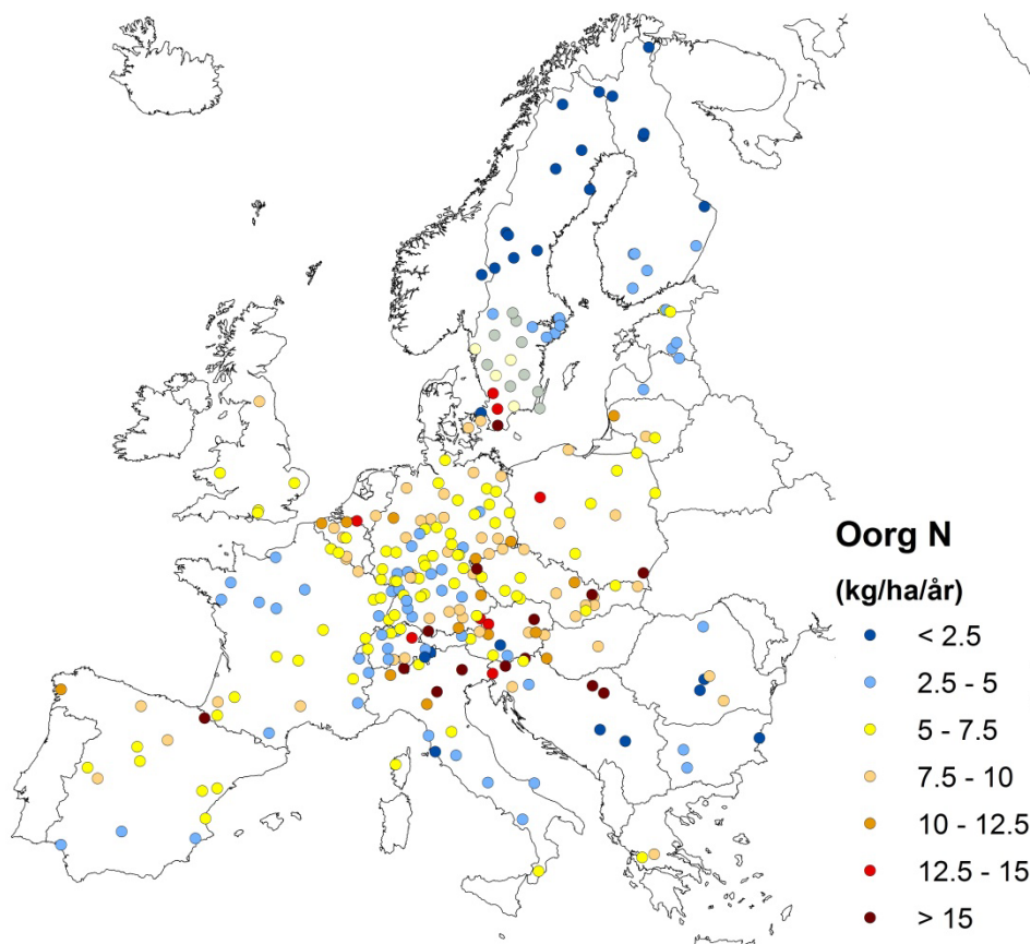
Figur 6. Nedfall av oorganiskt kväve ( \text{NO}_3 + \text{NH}_4 ) till öppet fält i Europa, medelvärden för kalenderåren 2014 och 2015. Data utanför Sverige kommer från ICP Forest, en verksamhet inom konventionen om gränsöverskridande luftföroreningar, CLRTAP. I de flesta fall ligger provtagningen på öppet fält belägen i ett skogslandskap.
