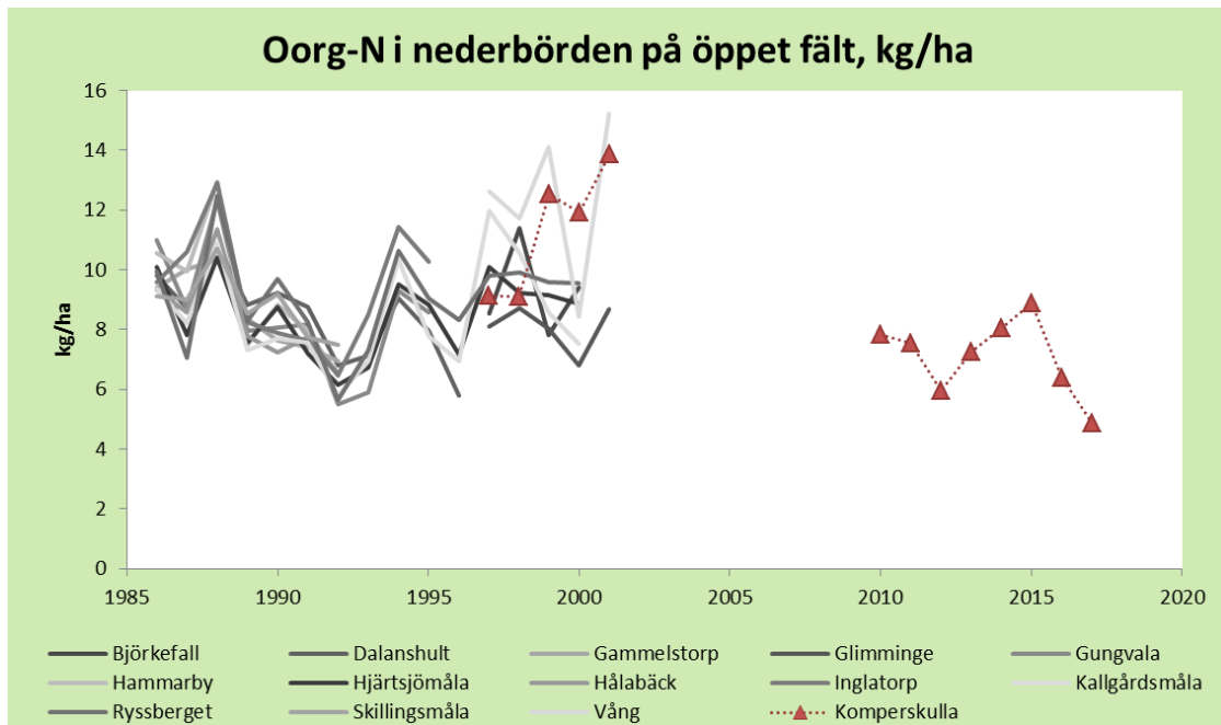
Figur 3. Nedfall av oorganiskt kväve (nitrat och ammonium) över öppet fält, vid samtliga ytor i länet inom Krondroppsnetet sedan 1985. Nedfallet mäts månadsvis och summeras för hydrologiskt år. Aktiva mätplatser visas med färgade symboler och avslutade mätplatser visas med linjer i grått och svart.
