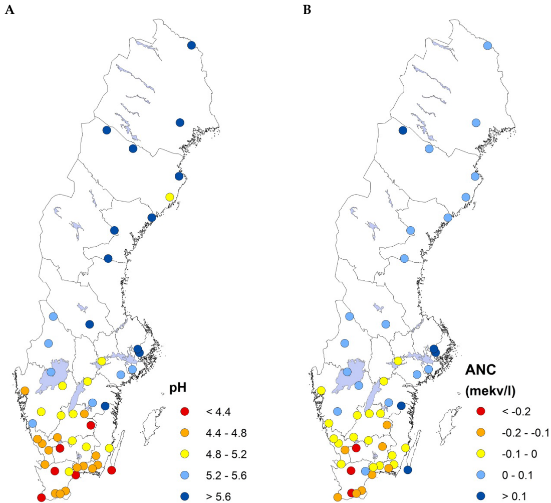
Figur 17. pH (A) och ANC (B) i markvattnet på 50 cm djup vid olika platser inom Krondroppsnetet. Det värde som anges är medianvärdet under de senaste tre åren (2015-2017). ANC i avrinnande vattnet bör vara betydligt över 0 när det når vattendragen. Ytor med mindre än 3 mätvärden under treårsperioden, samt ytor som har avverkats eller gödslats har tagits bort.
