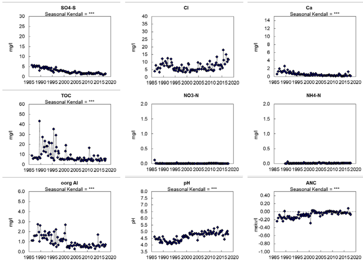
Figur B1.2. Markvattenkemi vid Hjartsjömåla, K 03: sulfatsvavel ( \text{SO}_4\text{-S} ), klorid ( \text{Cl}^- ), kalciumhalt ( \text{Ca}^{2+} ), totalt organiskt kol (TOC), nitratkväve ( \text{NO}_3\text{-N} ), ammoniumkväve ( \text{NH}_4\text{-N} ), oorganiskt aluminium (oorg Al), pH och markvattnets syraneutraliserande förmåga (ANC). Saknade värden innebär oftast att marken varit för torr. Trendanalys har genomförts med Seasonal-Kendall och signifikansnivåer anges, ovanför respektive diagram, i de fall där signifikanta trender påvisats.
