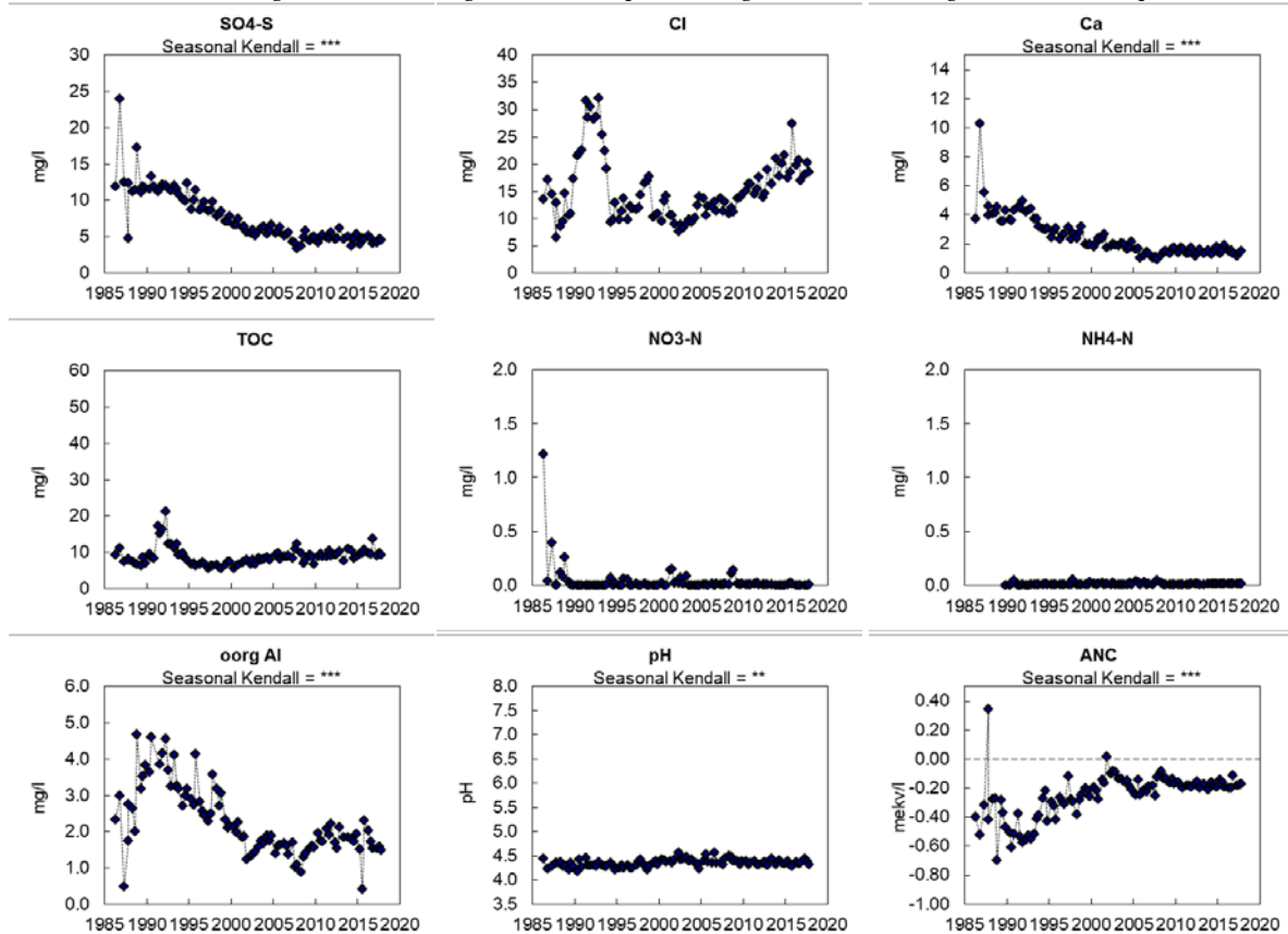
Figur B1.4. Markvattenkemi vid Ryssberget, K 07: sulfatsvavel ( \text{SO}_4\text{-S} ), klorid ( \text{Cl}^- ), kalciumhalt ( \text{Ca}^{2+} ), totalt organiskt kol (TOC), nitratkväve ( \text{NO}_3\text{-N} ), ammoniumkväve ( \text{NH}_4\text{-N} ), oorganiskt aluminium (oorg Al), pH och markvattnets syraneutraliserande förmåga (ANC). Saknade värden innebär oftast att marken varit för torr. Trendanalys har genomförts med Seasonal-Kendall och signifikansnivåer anges, ovanför respektive diagram, i de fall där signifikanta trender påvisats.
