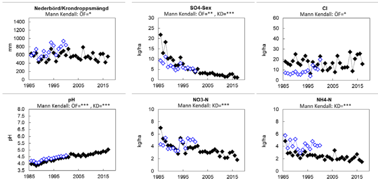
Figur B1.1. Årliga värden (hydrologiskt år) för depositionen via krondropp och över öppet fält vid Hjartsjömåla, K 03. I figuren visas uppmätt nederbörd över öppet fält samt krondroppsmängder sedan mätstart. Vidare redovisas nederbördens och krondroppets pH, liksom deposition för ett urval av ämnen: sulfatsvavel utan havssaltsbidrag ( \text{SO}_4\text{-S ex} ), klorid ( \text{Cl}^- ), nitratkväve ( \text{NO}_3\text{-N} ) och ammoniumkväve ( \text{NH}_4\text{-N} ). Trendanalys har genomförts med Mann-Kendall-analys. Signifikansnivåer anges, ovanför respektive diagram, i de fall där signifikanta trender påvisats.
