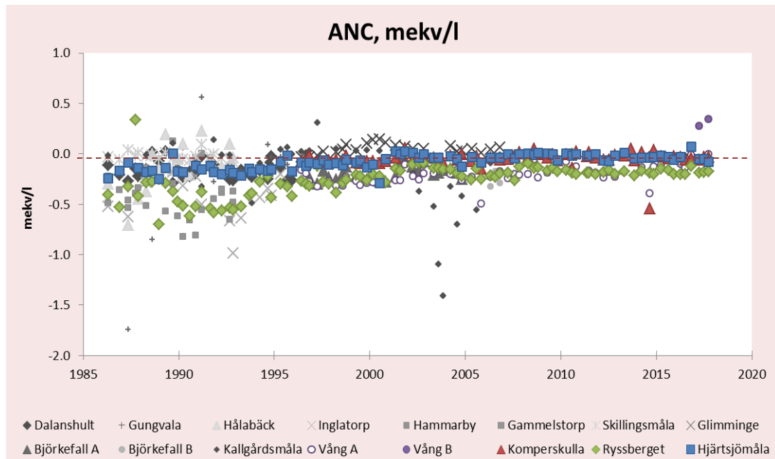
Figur 15. En sammanställning av alla förekommande mätningar av ANC i markvattnet i länet. Markvattnet provtas normalt tre gånger årligen, före, under och efter växtsäsongen. Vid vissa tillfällen saknas prov när det varit torrt i marken. Aktiva mätplatser visas med färgade symboler och avslutade mätplatser visas med symboler i grått och svart.
