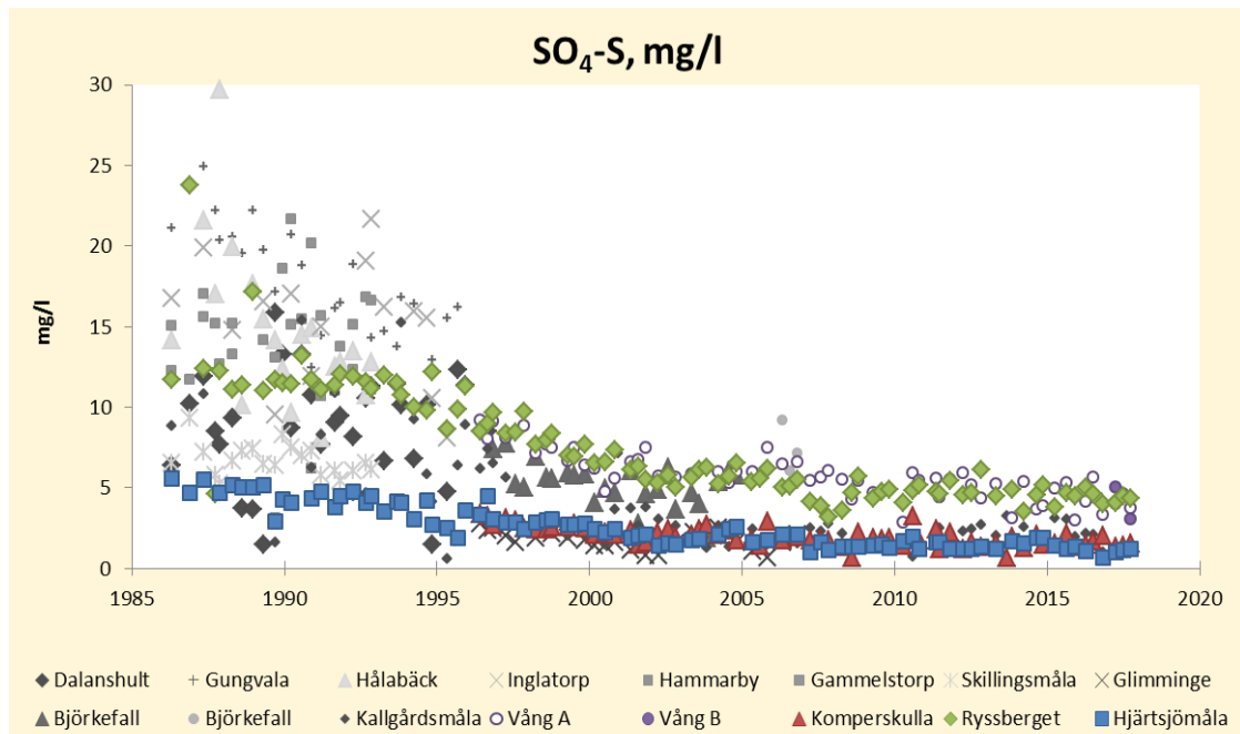
Figur 13. En sammanställning av alla förekommande mätningar av svavelhalter i markvattnet i länet. Markvattnet provtas normalt tre gånger årligen, före, under och efter växtsäsongen. Vid vissa tillfällen saknas prov när det varit torrt i marken. Aktiva mätplatser visas med färgade symboler och avslutade mätplatser visas med symboler i grått och svart.
