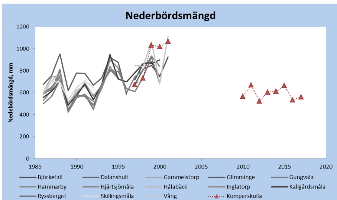
Figur 4. Nederbördsmängd (mm) vid samtliga mätningar på öppet fält i Blekinge län sedan mätstarten 1985. Nedfallet mäts månadsvis och summeras för hydrologiskt år. Aktiva mätplatser visas med färgade symboler och avslutade mätplatser visas med linjer i grått och svart.
