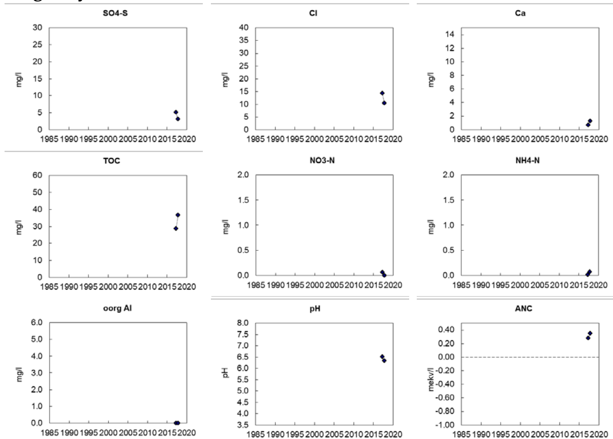
Figur B1.10. Markvattenkemi vid Vång, K 13B: sulfatsvavel ( \text{SO}_4\text{-S} ), klorid ( \text{Cl} ), kalciumhalt ( \text{Ca}^{2+} ), totalt organiskt kol (TOC), nitratkväve ( \text{NO}_3\text{-N} ), ammoniumkväve ( \text{NH}_4\text{-N} ), oorganiskt aluminium (oorg Al), pH och markvattnets syraneutraliserande förmåga (ANC). Saknade värden innebär oftast att marken varit för torr. Trendanalys har genomförts med Seasonal-Kendall och signifikansnivåer anges, ovanför respektive diagram, i de fall där signifikanta trender påvisats.
