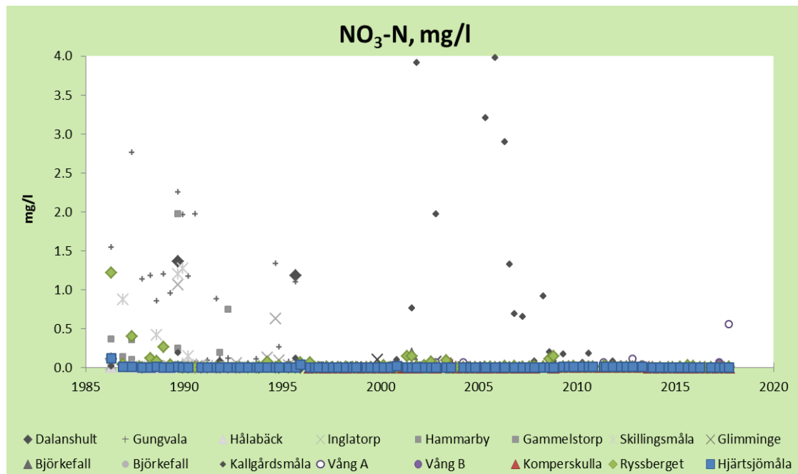
Figur 7. Nitrathalter i markvattnet vid samtliga ytor inom Krondroppsnetet sedan 1986. I Kallgårdsmåla gick nitratkvävehalten upp till 25 mg/l hösten 2003 som en effekt av avverkning, men detta visas inte i figuren eftersom en anpassning av y-skalan till Kallgårdsmåla skulle innebära att variationer på andra ytor skulle vara svårare att se. Aktiva mätplatser visas med färgade symboler och avslutade mätplatser visas med symboler i grått och svart.
