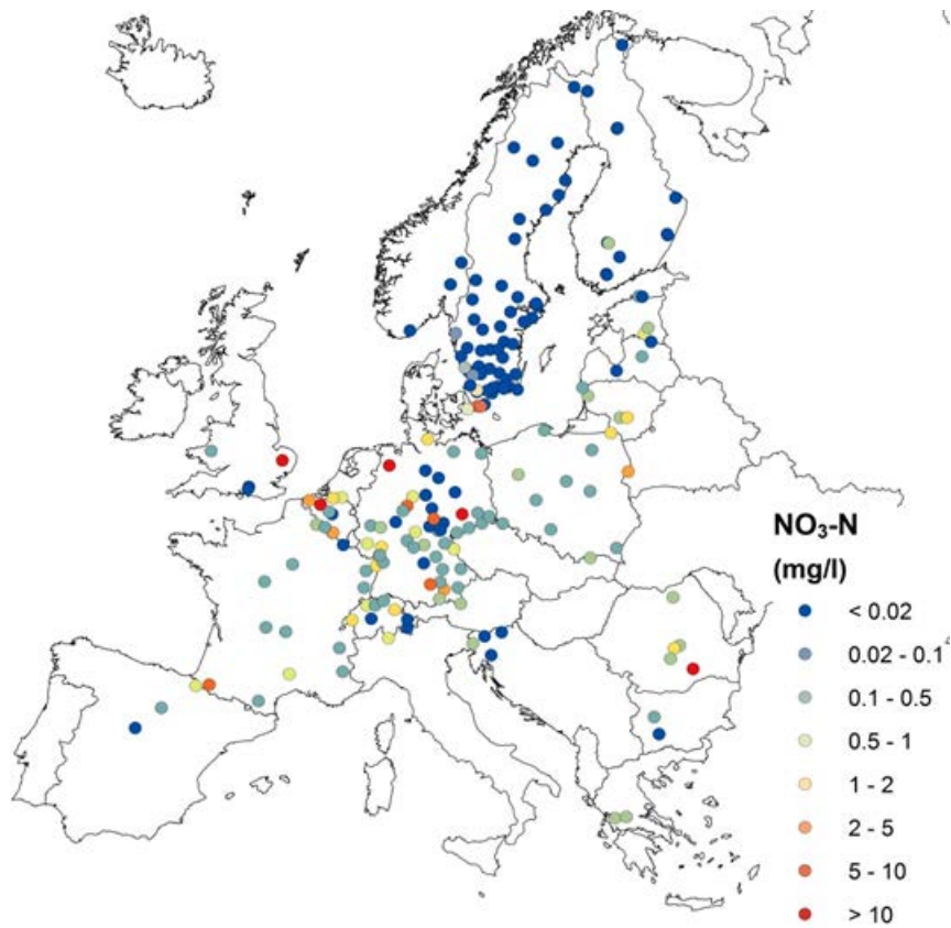
Figur. 9. Koncentrationen av nitrat (NO 3 -N) i markvattnet (median för 3 mätningar/år under 2014-2016, 50 cm djup) vid olika platser inom Krondroppsnetet, samt ICP-Forestdata (median för månadsvärden under 2014-2016, 40-80 cm djup). Observera att skalan är en annan än i Figur 8.
