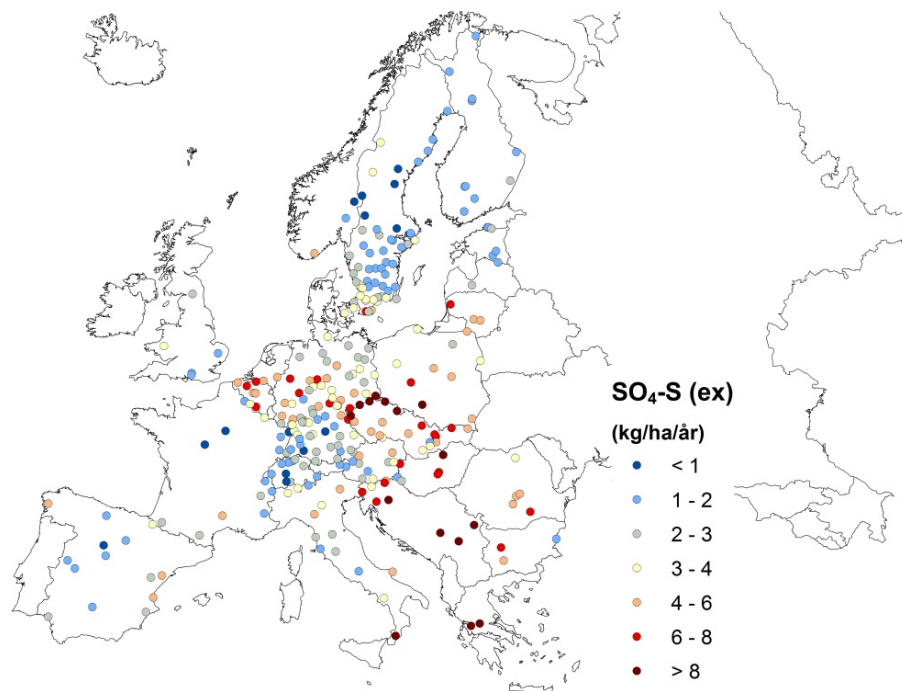
Figur 12. Årligt svavelnedfall till skog som krondropp som medelvärde för de två kalenderåren 2014-2015 vid provytor med varierande trädslag inom ICP Forest, en verksamhet inom konventionen om långväga transporterade luftföroreningar, LRTAP. Notera att skalan inte är den samma som i Figur 11.
